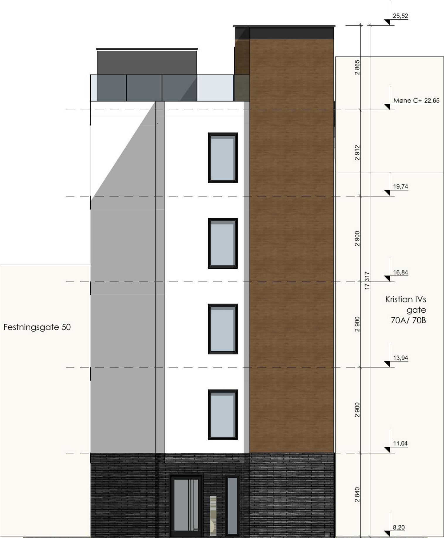
Sørøst fasade
